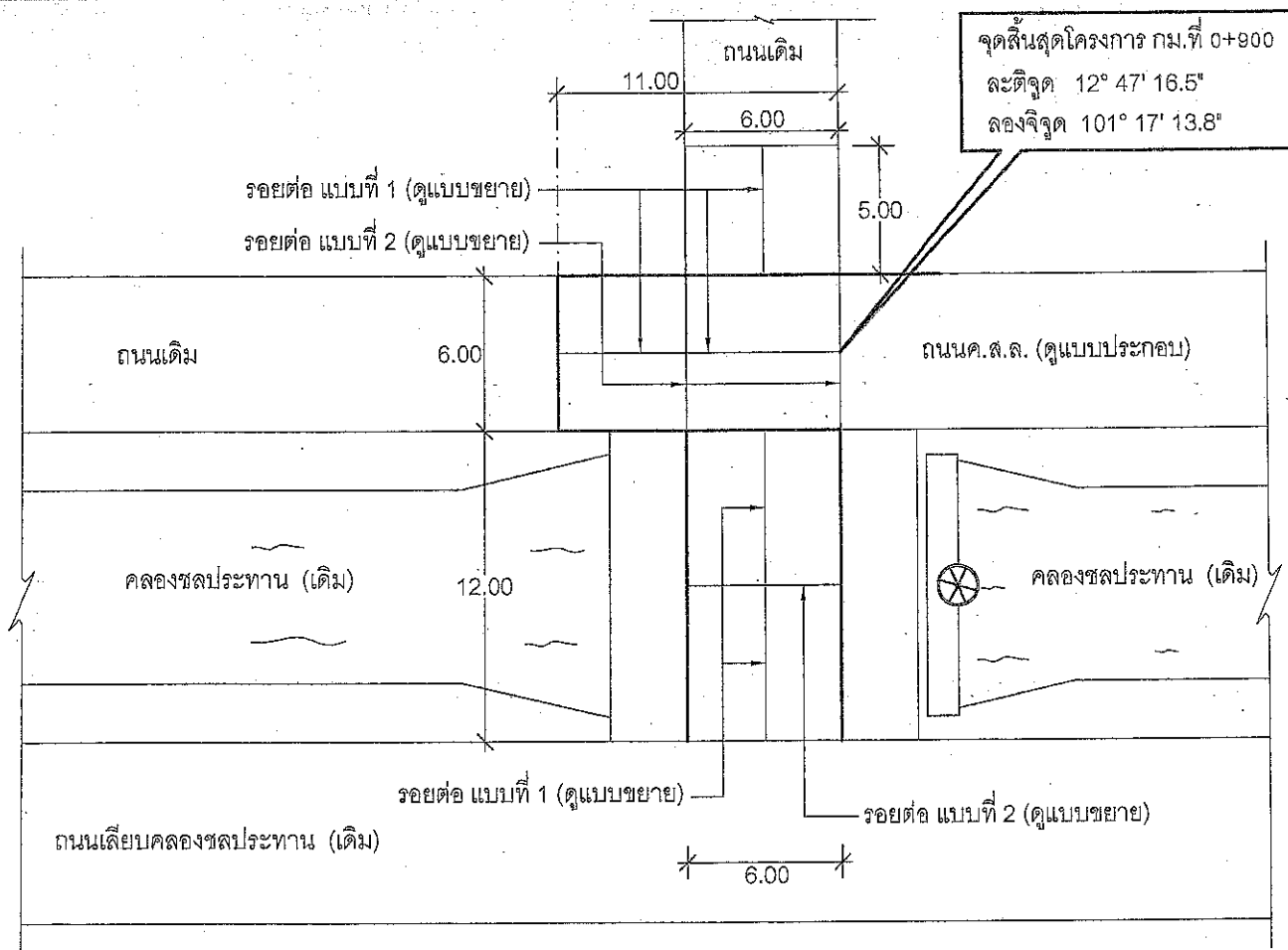
แปลนขยายจุดเชื่อมต่อถนน ค.ส.ล. NOT TO SCALE
