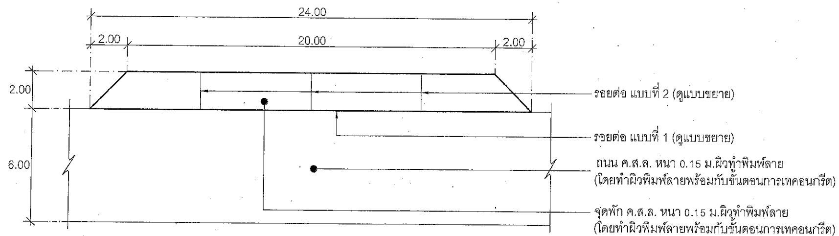
แปลนขยายจุดพัก ค.ส.ล. จุดที่ 3 NOT TO SCALE
