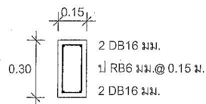
ขยาย GB NOT TO SCALE
