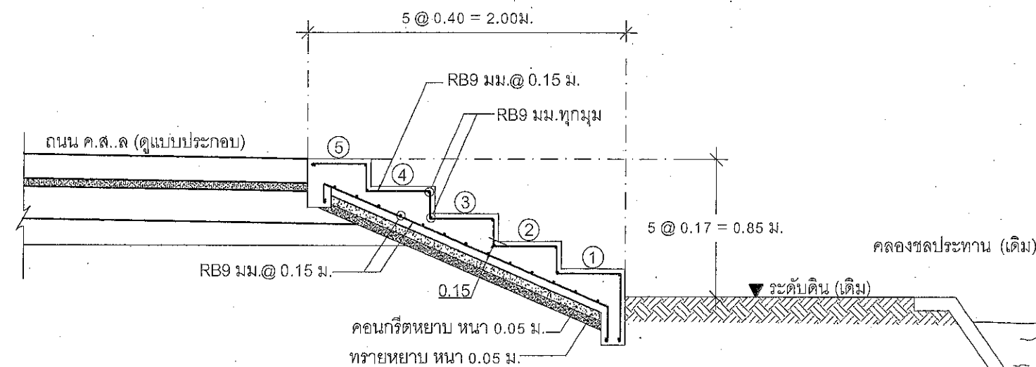
รูปตัดบันได ค.ส.ล. NOT TO SCALE
