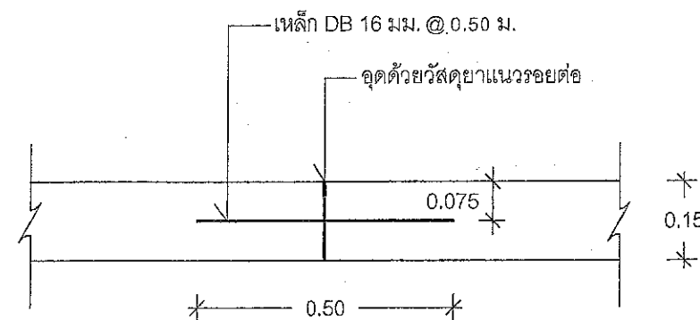
LONGITUDINAL JOINT
