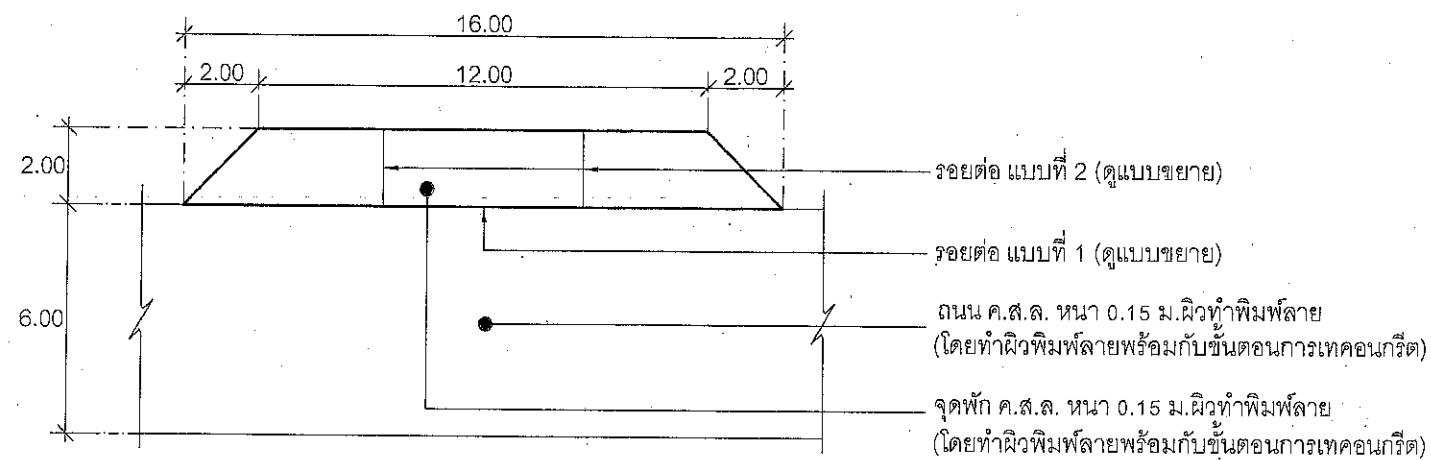
แปลนขยายจุดพัก ค.ส.ล. จุดที่ 1, จุดพัก ค.ส.ล. จุดที่ 2, จุดพัก ค.ส.ล. จุดที่ 4 และ จุดพัก ค.ส.ล. จุดที่ 5 NOT TO SCALE
