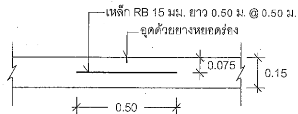
แบบขยายรอยต่อแบบที่ 2 จุดพัก ค.ส.ล.จุดที่ 1,จุดพัก ค.ส.ล.จุดที่ 2,จุดพัก ค.ส.ล.จุดที่ 3,จุดพัก ค.ส.ล.จุดที่ 4 และ จุดพัก ค.ส.ล.จุดที่ 5 NOT TO SCALE
