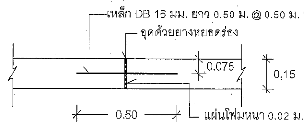
แบบขยายรอยต่อแบบที่ 1 จุดพัก ค.ส.ล.จุดที่ 1,จุดพัก ค.ส.ล.จุดที่ 2,จุดพัก ค.ส.ล.จุดที่ 3,จุดพัก ค.ส.ล.จุดที่ 4 และ จุดพัก ค.ส.ล.จุดที่ 5 NOT TO SCALE
