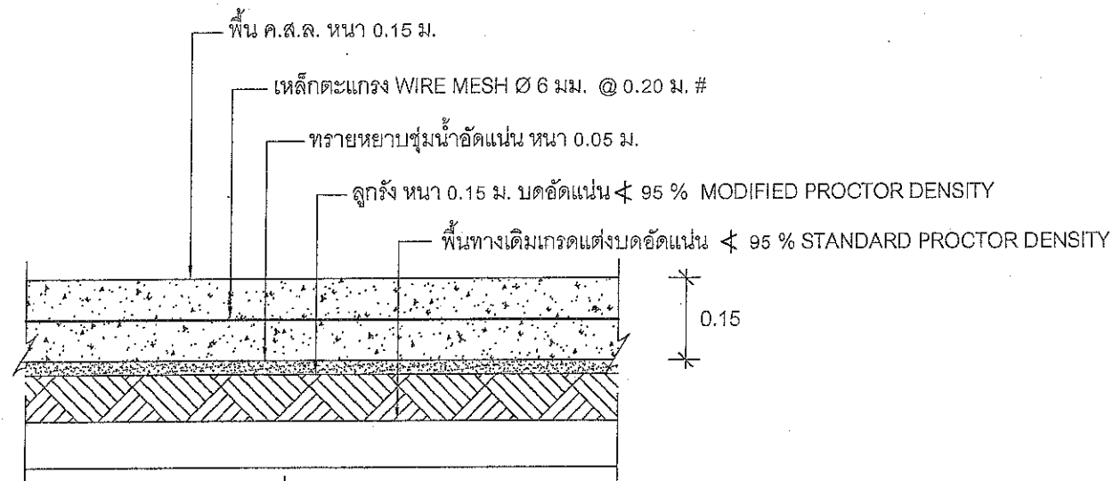
รูปตัดจุดเชื่อมต่อถนน ค.ส.ล.
