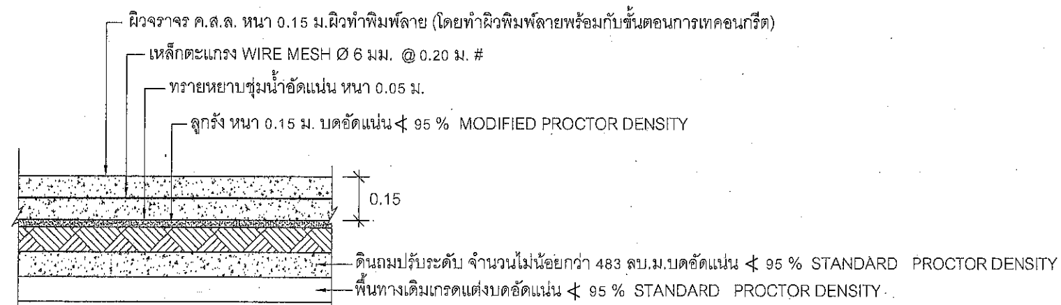
รูปตัดจุดพัก ค.ส.ล.จุดที่ 1,จุดพัก ค.ส.ล.จุดที่ 2,จุดพัก ค.ส.ล.จุดที่ 3,จุดพัก ค.ส.ล.จุดที่ 4 และ จุดพัก ค.ส.ล.จุดที่ 5 NOT TO SCALE
