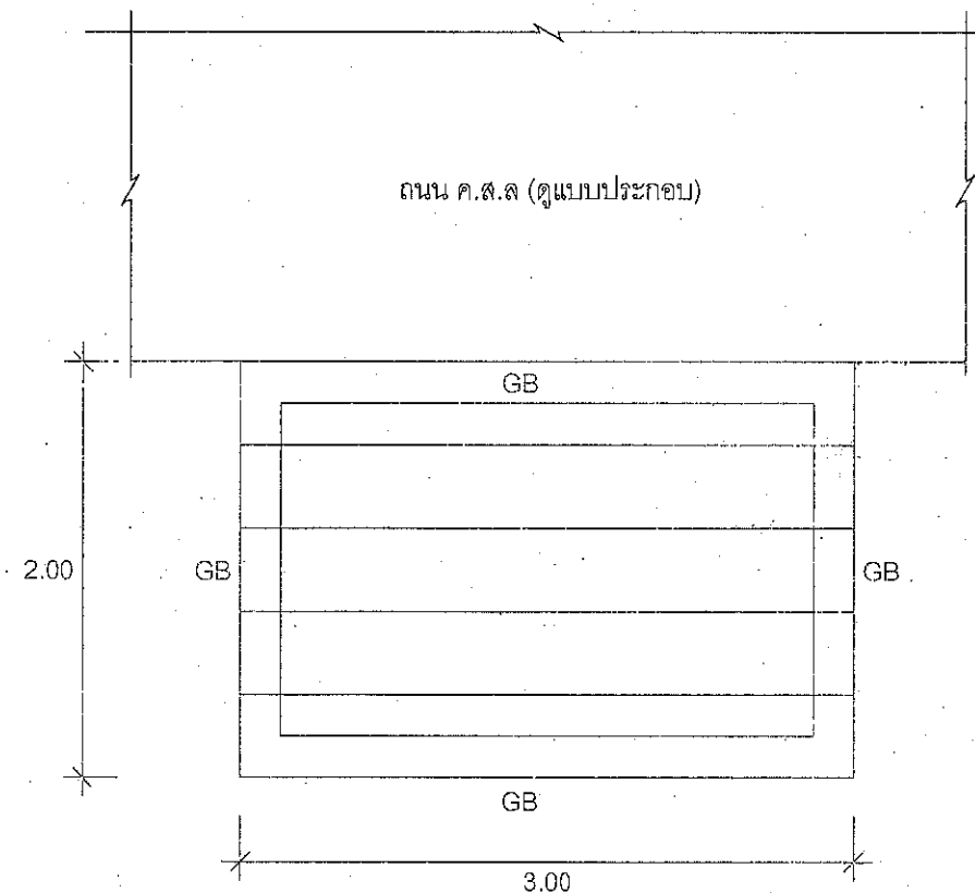
แปลนคานบันได ค.ส.ล. SCALE : 100
