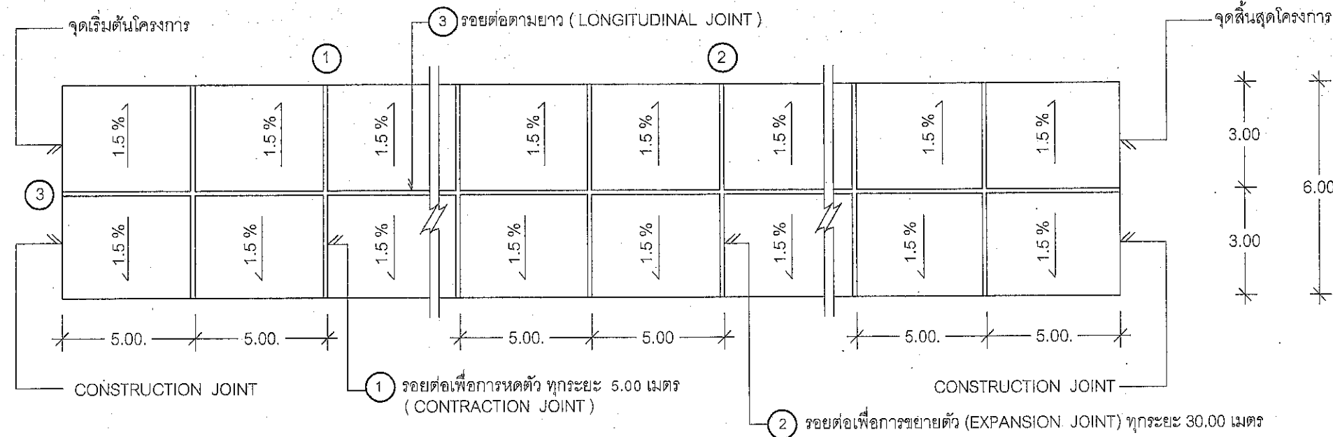
แปลนพื้นถนน ค.ส.ล. NOT TO SCALE
