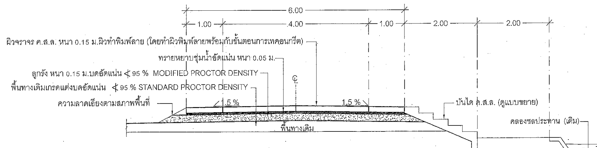
รูปตัด ก ถนน ค.ส.ล. (แบบมีจุดพัก ค.ส.ล.) NOT TO SCALE
