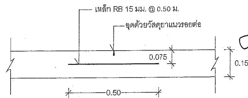
ขยายรอยต่อ แบบที่ 2 (จุดเชื่อมต่อถนน ค.ส.ล.)
