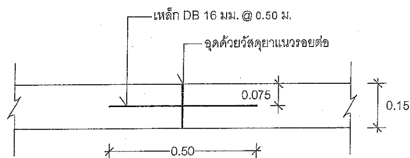
ขยายรอยต่อ แบบที่ 1 (จุดเชื่อมต่อถนน ค.ส.ล.)
