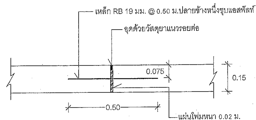
ขยายรอยต่อสำหรับหยุดก่อสร้าง (จุดเชื่อมต่อถนน ค.ส.ล.)
